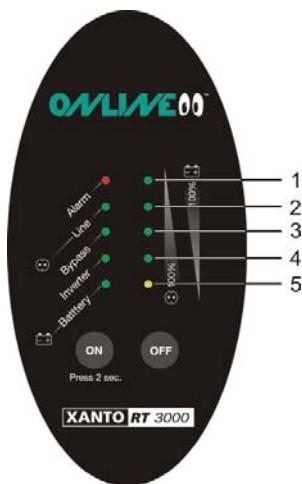
Figura 2: Comandi e indicatori
