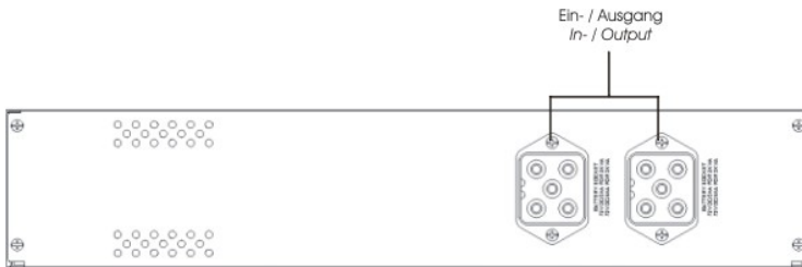
Abbildung 7: Rückseite XANTO RT Batteriepaket
