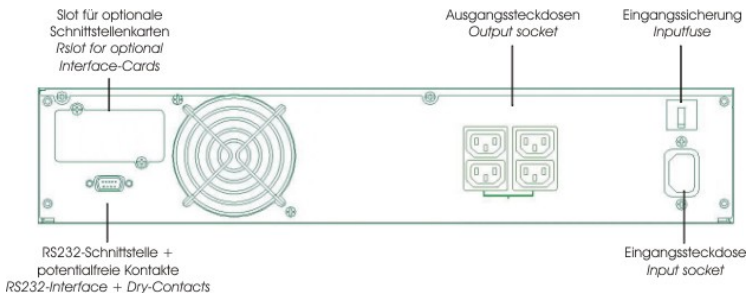
Abbildung 3: Rückseite XANTO RT 1000
