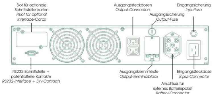
Figura 5: Pannello posteriore del sistema XANTO RT 3000
