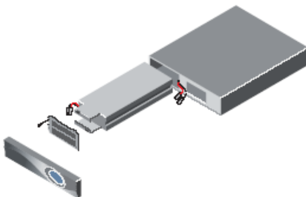
Figura 13: Batterie hot-swap nel modello XANTO RT 1000
