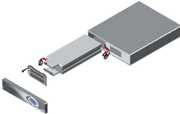
Abbildung 13: Hot-Swap-Batterie bei XANTO RT 1000
