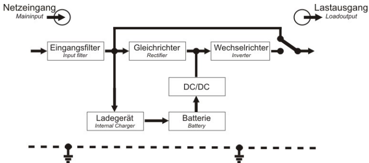
Figura 8: Schema elettrico a blocchi
