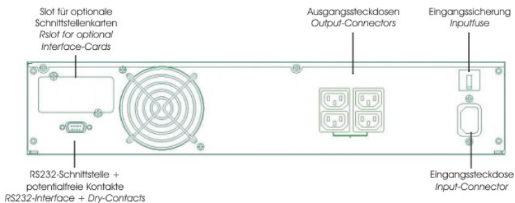
Figura 3: Pannello posteriore del sistema XANTO RT 1000
