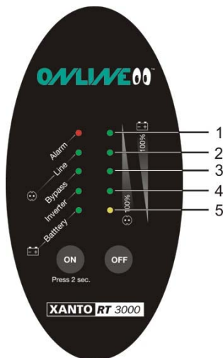
Abbildung 2: Bedien- und Anzeigeelemente
