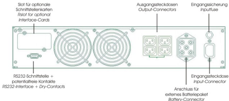
Figura 4: Pannello posteriore del sistema XANTO RT 2000
